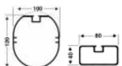
LATTE/PFOSTEN BODENRAHMEN
