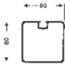
LATTE/PFOSTEN BODENRAHMEN
